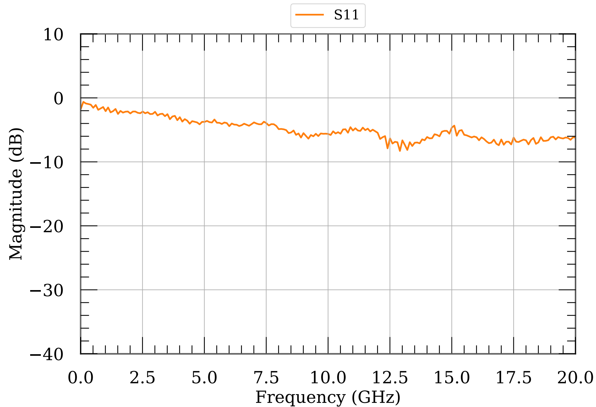
LNA S-params module004
